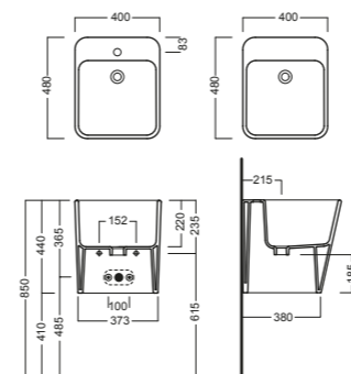
PILOZZO SOSPESO 480x400x440h
